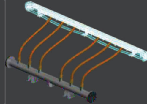
PROTEÇÃO CONTRA TRANSBORDAMENTO DE LODO (CURB FIXO)
