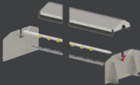
CHUVEIRO DE LIMPEZA DO TECIDO FILTRANTE
