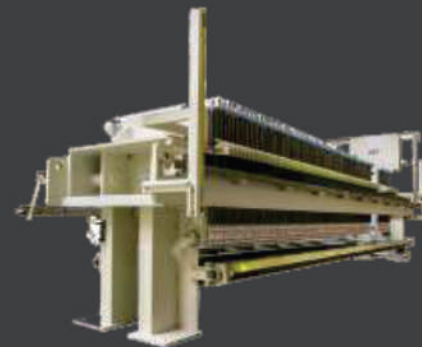
FILTRO PRENSA
